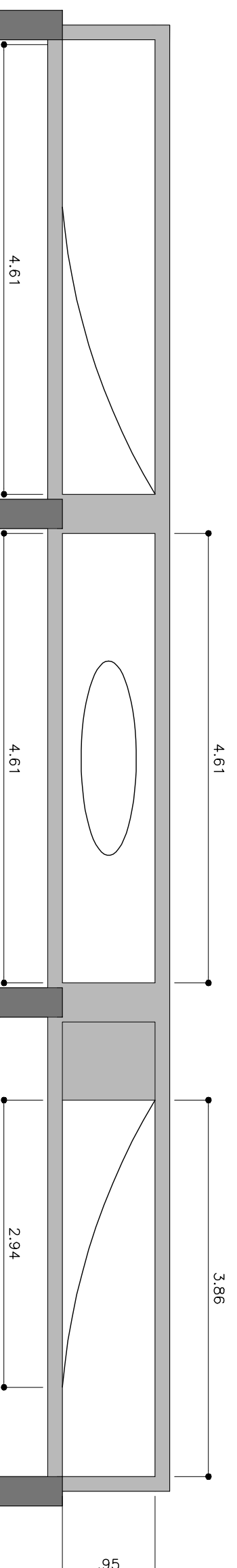
PLANTA BAIXA - LAYOUT E COTAS JARDIM HALL DE ENTRADA esc.: 1/50
